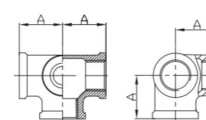
Side Outlet Tee
